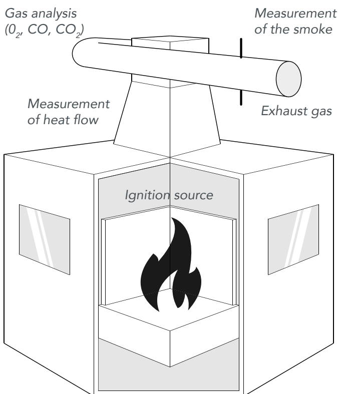
SBI test
